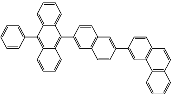
(2-72)
