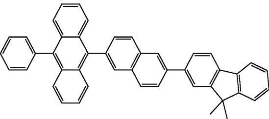
(2-74)
