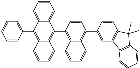
(2-73)
