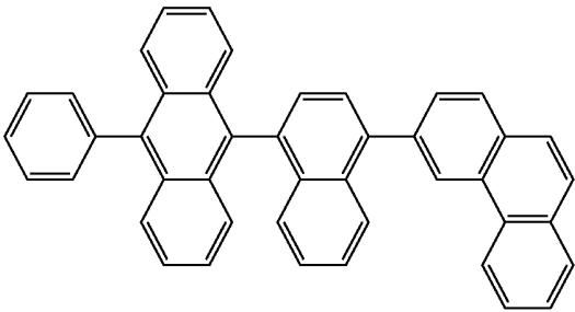
(2-70)
