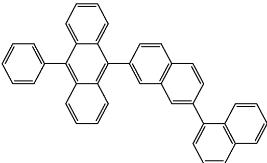
(2-63)
