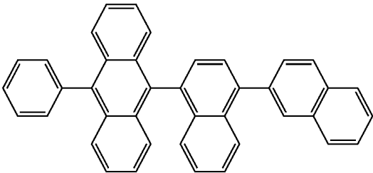
(2-66)
