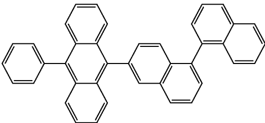
(2-64)
