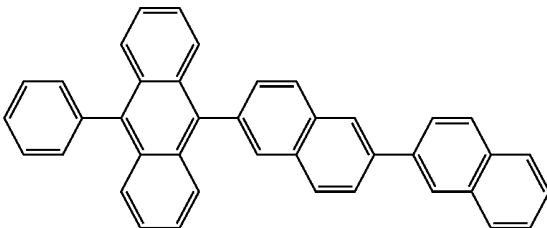
(2-62)
