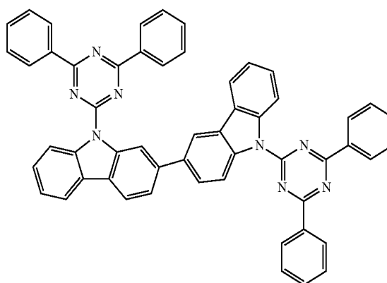
(1-104)
