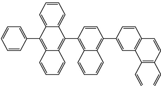
(2-69)
