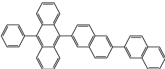
(2-69)
