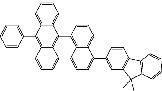
(2-74)
