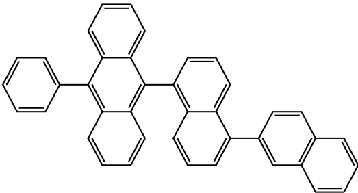
(2-57)
