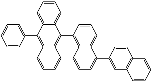
(2-67)
